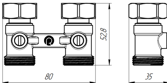
Рисунок 1 – Размеры клапана (узла) нижнего подключения KYR01
