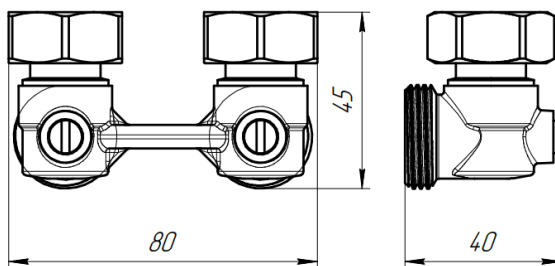
Рисунок 2 – Размеры клапана (узла) нижнего подключения KYR02
